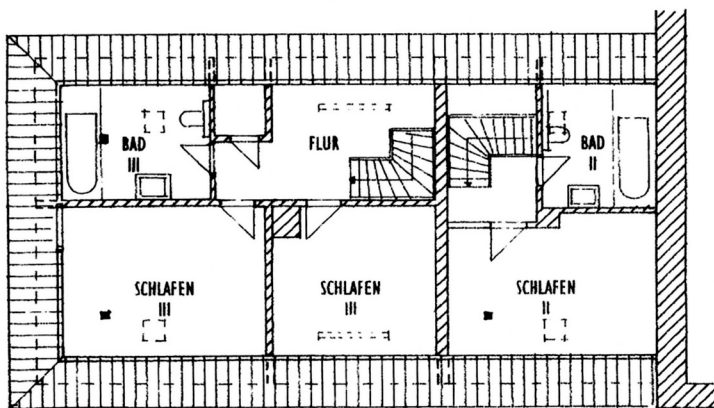
Herrenhaus, linker Seitenflügel, Dachgeschoß
