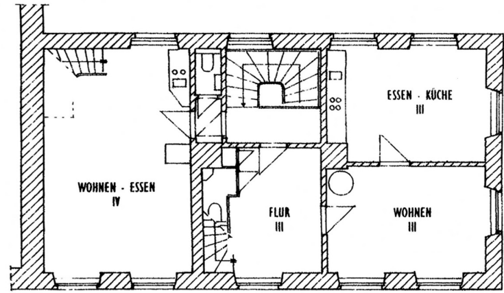
rechter Seitenflügel, I. OG
