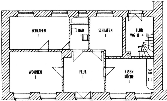
Herrenhaus, linker Seitenflügel, Erdgeschoß
