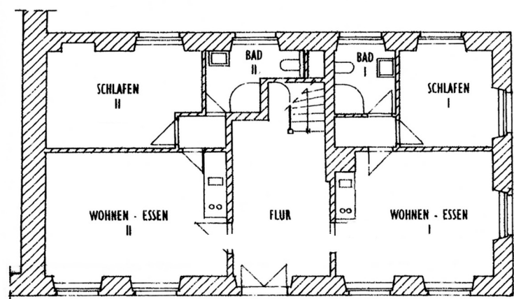
rechter Seitenflügel, Erdgeschoß
